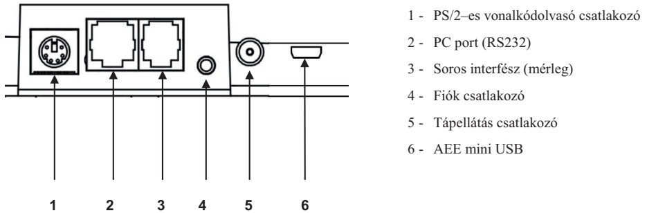
2. ábra - Csatlakozók a pénztárgép alján
